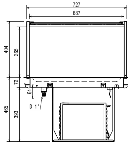
Front aanzicht
